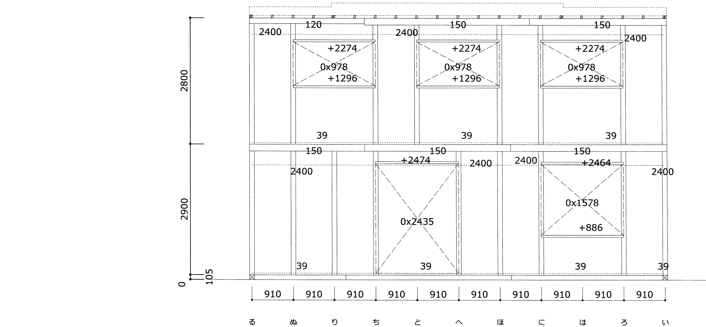
10通り 南面
