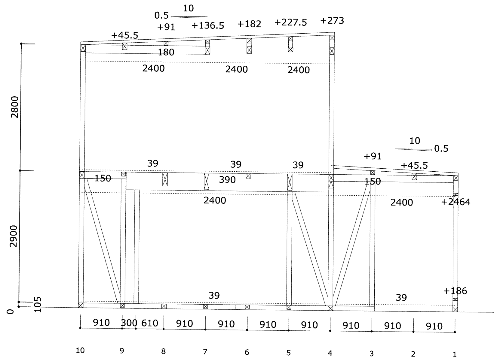
ほ通り 東面
