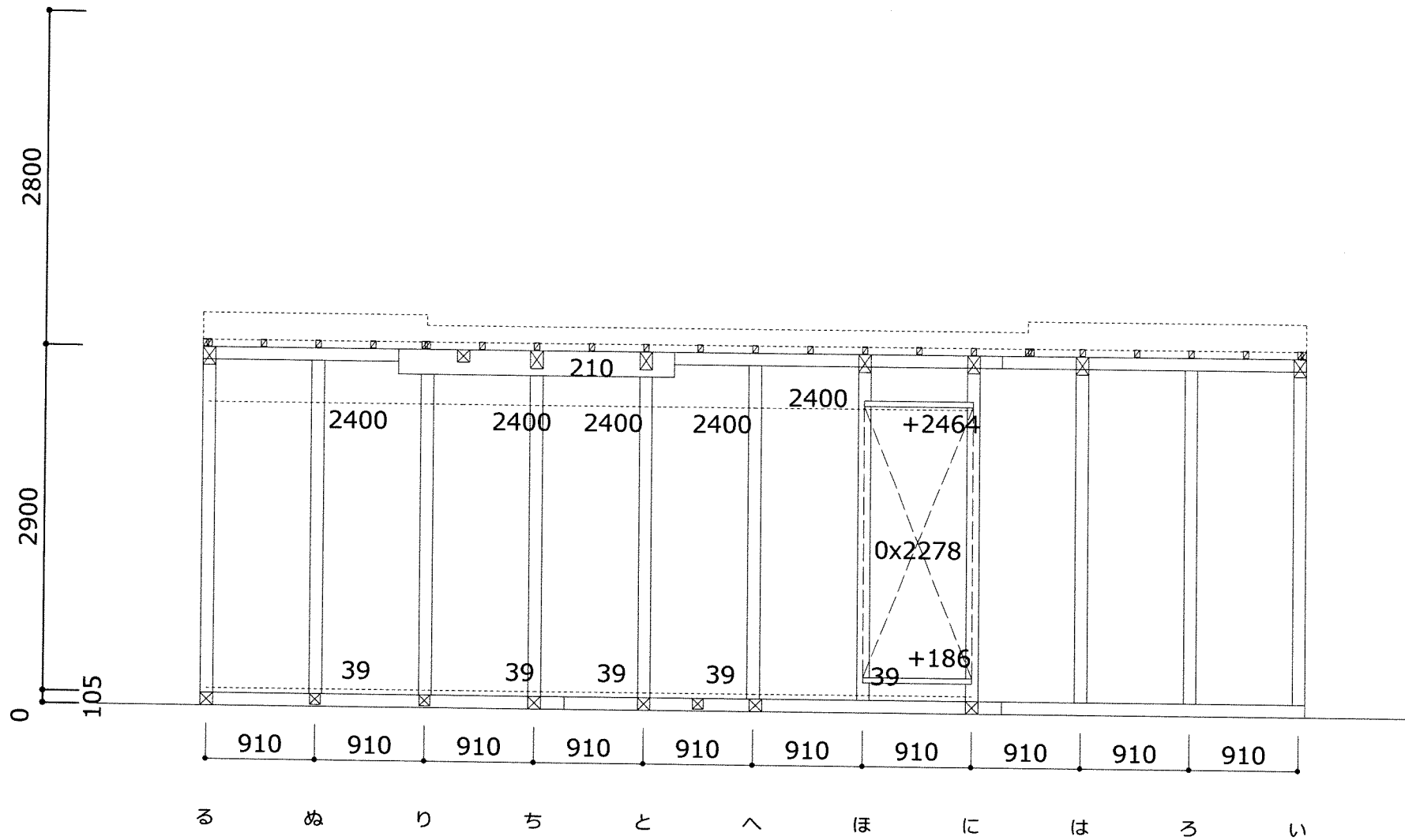
1通り 南面
